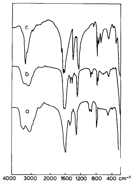
Fig. 5. IR spectra of (a) (\text{CH}_3\text{NH}_3)_2\text{Cd}(\text{C}_2\text{O}_4)_2(\text{CH}_3\text{NH}_3) \cdot \text{H}_2\text{O} ; (b) (\text{CH}_3\text{NH}_3)_2\text{Mn}_2(\text{C}_2\text{O}_4)_3(\text{CH}_3\text{NH}_2) \cdot \text{H}_2\text{O} ; and (c) \text{Cu}(\text{C}_2\text{O}_4)(\text{NH}_3)_2 \cdot 2\text{H}_2\text{O} .
