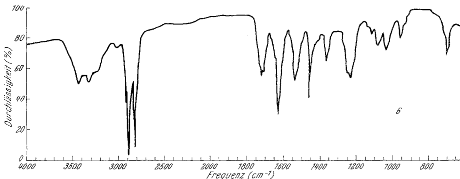
Abb. 4. IR-Spektrum der Verbindung 6
