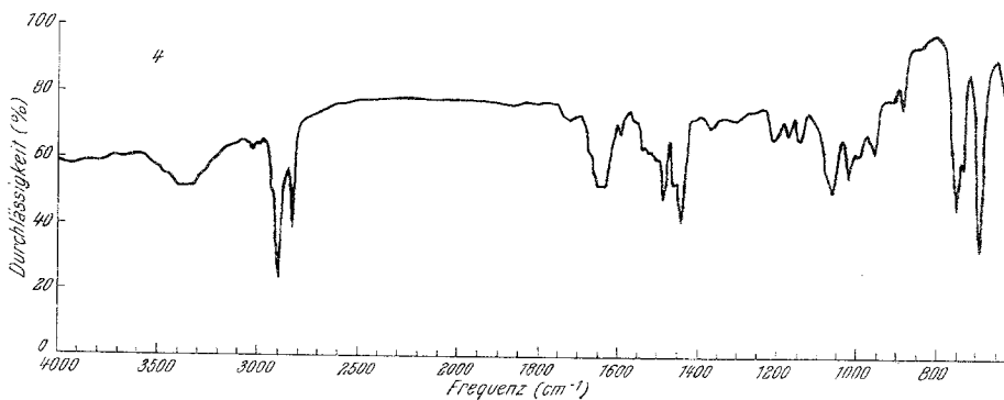
Abb. 3. IR-Spektrum der Verbindung 4
