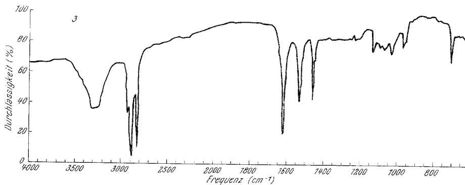
Abb. 2. IR-Spektrum der Verbindung 3
