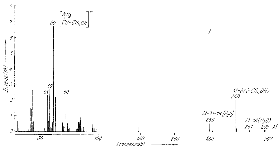
Abb. 1. Massenspektrum der Verbindung 2
