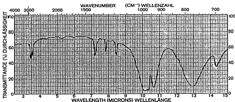
Fig. 2. IR-Spektrum von (\text{CH}_3)_3\text{SnO}_2\text{SCH}_3 ( 670\text{--}4000\text{ cm}^{-1} , fest/KBr).
