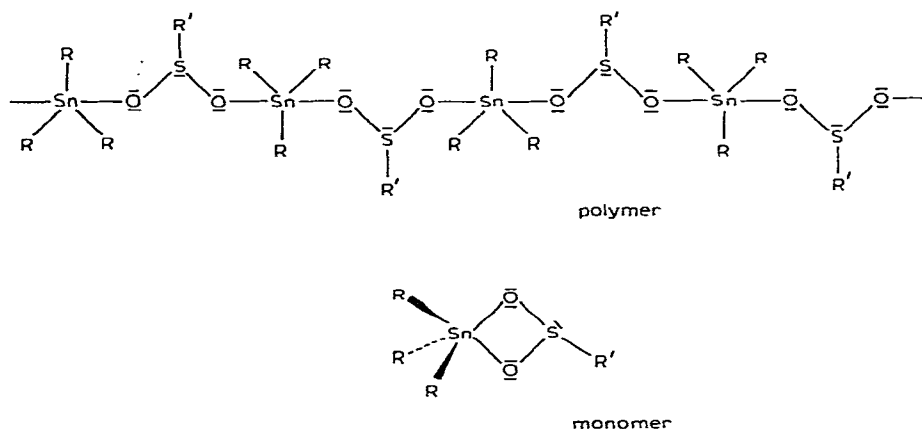
Fig. 1. Mögliche Strukturmodelle für Trialkylzinn-alkansulfonate, \text{R}_3\text{SnO}_2\text{SR} ( \text{R} = \text{CH}_3, \text{C}_2\text{H}_5, \text{n-C}_3\text{H}_7, \text{i-C}_3\text{H}_7, \text{n-C}_4\text{H}_9 ).
