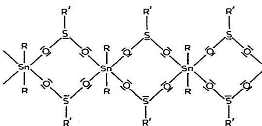
Fig. 3. Strukturmodell für Diorganozinn-bis(sulfinate), \text{R}_2\text{Sn}(\text{O}_2\text{SR})_2 ( \text{R} = \text{CH}_3, \text{C}_2\text{H}_5, n\text{-C}_3\text{H}_7, i\text{-C}_3\text{H}_7, n\text{-C}_4\text{H}_9 ).
