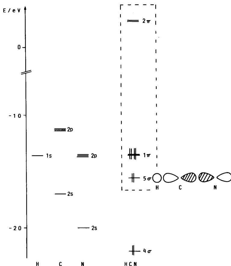
Fig. 1. Halbquantitatives (Grenz-) Molekülorbital-Schema von HCN.
