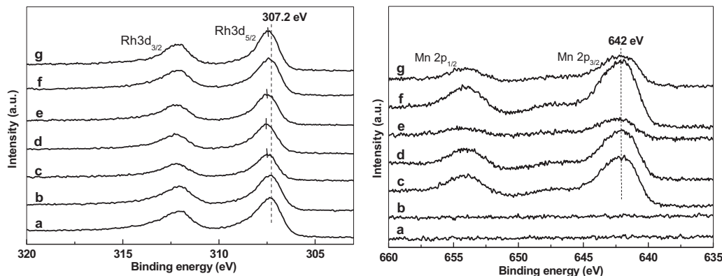
Fig. 2. XPS spectra of samples: (a) 1.5Rh/ SiO_2 ; (b) 1.5Rh-0.075Li/ SiO_2 ; (c) 1.5Rh-1.5Mn/ SiO_2 ; (d) 1.5Rh-1.5Mn-0.075Li/ SiO_2 ; (e) 1.5Rh-0.5Mn-0.075Li/ SiO_2 ; (f) 1.5Rh-2.5Mn-0.075Li/ SiO_2 ; (g) 1.5Rh-1.5Mn-0.45Li/ SiO_2 .
