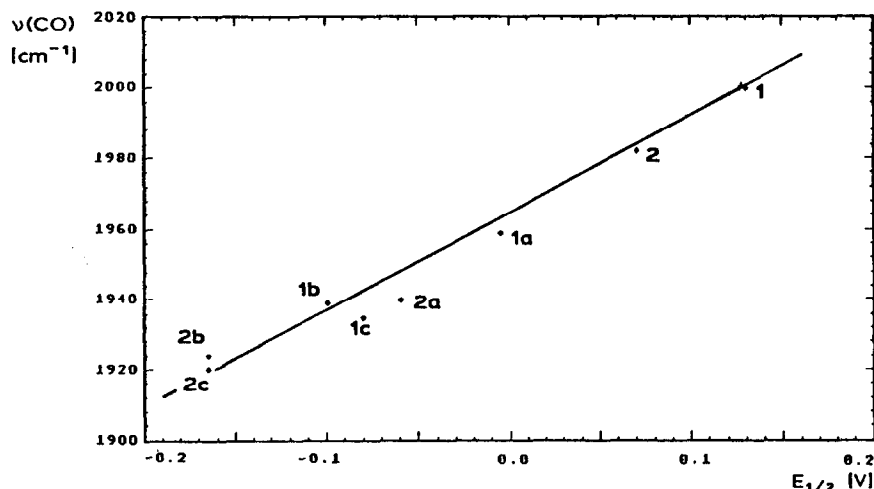
Fig. 1. Korrelation zwischen Redoxpotential E_{1/2} (in \text{CH}_2\text{Cl}_2 ) und Valenzfrequenz \nu(\text{CO}) (in Hexan). (Für die Dicarbonylkomplexe 1 und 2 wurden die Mittelwerte der beiden Schwingungsabsorptionen der Rasse A und B verwendet).
