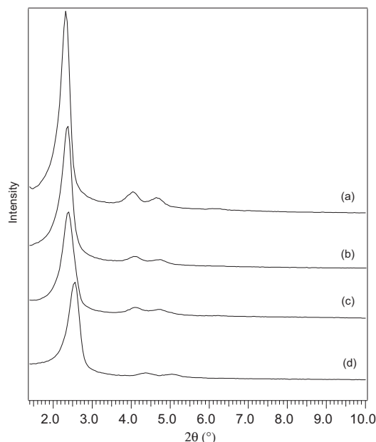
Fig. 3. The low angle XRD patterns of (a) MCM-41; (b) 5 wt.% TPA/MCM-41, (c) 10 wt.% TPA/MCM-41, (d) 15 wt.% TPA/MCM-41.
