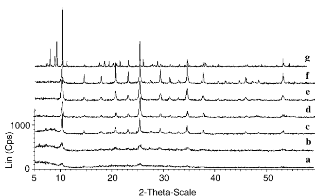
Figure 4. XRD patterns for a) TPA 23 /SBA-15v, b) TPA 46 /SBA-15v, c) TPA 60 /SBA-15v, d) TPA 67 /SBA-15v, e) TPA 73 /SBA-15v, f) TPA 78 /SBA-15v, and g) bulk TPA.
