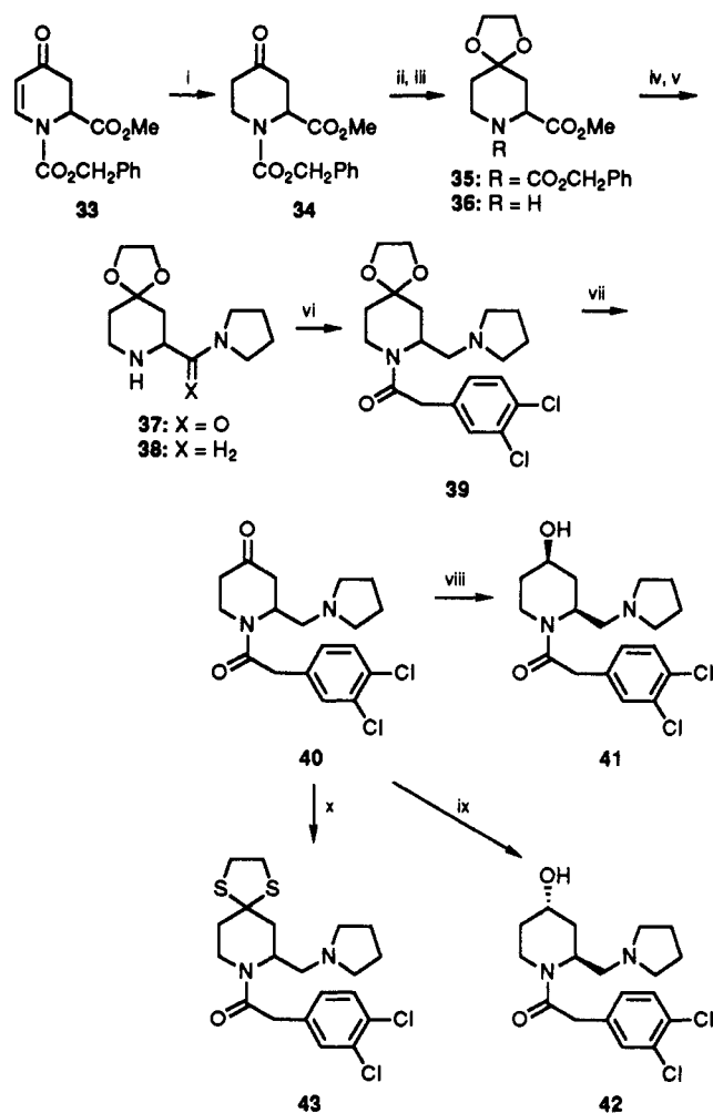
Scheme VI a
