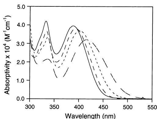
Fig. 3. UV-vis spectra of \text{Mo(CO)}_4(\text{Dmic})_2 (—), \text{Mo(CO)}_4(\text{Mic})_2 (---), \text{Mo(CO)}_4(\text{Cmic})_2 (-.-), and \text{Mo(CO)}_4(\text{Tic})_2 (---) in \text{CH}_2\text{Cl}_2 solution.
