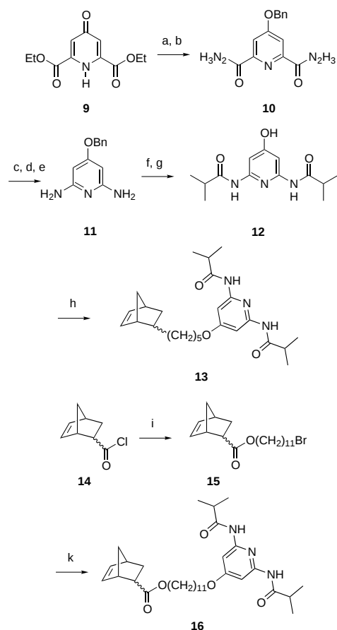
Scheme 4. Synthesis of diaminopyridine monomers 13 and 15 . a) BzBr, K 2 CO 3 , DMF, 80 °C, 4 h, 78 %. b) N 2 H 4 , EtOH, reflux, 12 h, 92 %. c) NaNO 2 , HCl, 0 °C, 20 min. d) EtOH, reflux, 12 h. e) EtOH/KOH (aq.), reflux, 18 h, 49 % (overall). f) isobutyl chloride, NEt 3 , DCM, 25 °C, 86 %. g) H 2 , Pd/C, EtOH, 100 %. h) 8 , K 2 CO 3 , DMSO, 90 °C, 4 h, 83 %. i) Bromoundecanol, pyridine, THF, reflux, 2 h, 91 %. k) 12 , K 2 CO 3 , DMSO, 90 °C, 4 h, 65 %.
