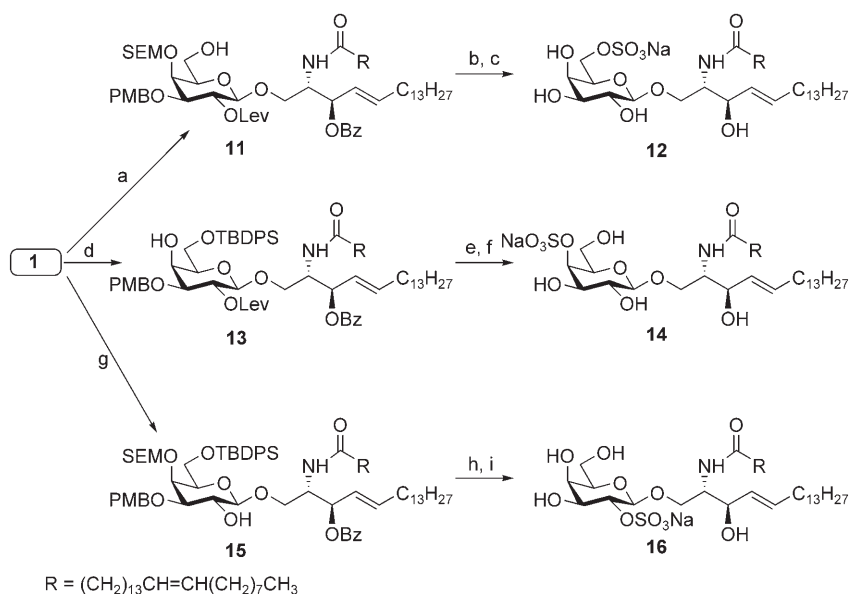
Scheme 3. a) TBAF, THF/AcOH, 86%; b) \text{SO}_3\cdot\text{Me}_3\text{N} , DMF, 40^{\circ}\text{C} , 73%; c) 1) \text{CF}_3\text{COOH} 5% in \text{CH}_2\text{Cl}_2 , 2) \text{MeONa} , \text{MeOH}/\text{CH}_2\text{Cl}_2 , 3) Dowex \text{Na}^+ form, 70%; d) \text{MgBr}_2 , \text{Et}_2\text{O}/\text{CH}_3\text{NO}_2 , 84%; e) \text{SO}_3\cdot\text{Me}_3\text{N} , DMF, 40^{\circ}\text{C} , 68%; f) 1) \text{CF}_3\text{COOH} 5% in \text{CH}_2\text{Cl}_2 , 2) TBAF, THF, 3) \text{MeONa} , \text{MeOH}/\text{CH}_2\text{Cl}_2 , 4) Dowex \text{Na}^+ form, 66%; g) \text{NH}_2\text{NH}_2\cdot\text{AcOH} , \text{CH}_2\text{Cl}_2/\text{MeOH} 82%; h) \text{SO}_3\cdot\text{Me}_3\text{N} , DMF, 40^{\circ}\text{C} , 62%; i) see f), 75%.
