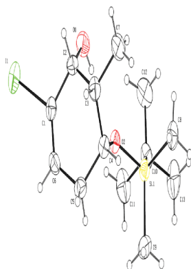
Fig. 2 ORTEP diagram of 13 .
