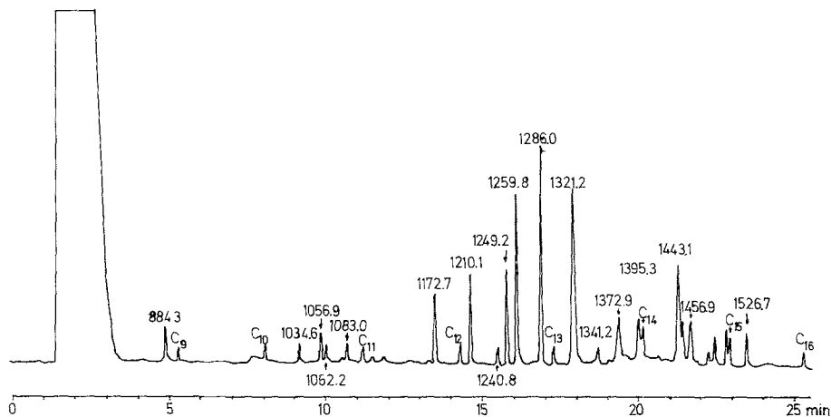
Abb. 3. Methylierte Säurefraktion aus dem Abbau des Hydroperoxids 4
