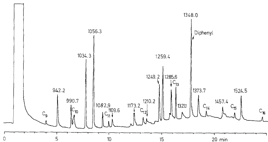
Abb. 4. Methylierte Säurefraktion aus dem Abbau des Kreosol 1 (90 °C, 10 bar O 2 , 90 min)
