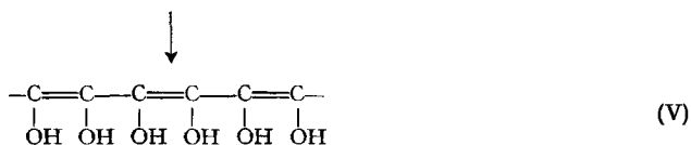
Schema 1 n \text{ HOC}\equiv\text{COH}
