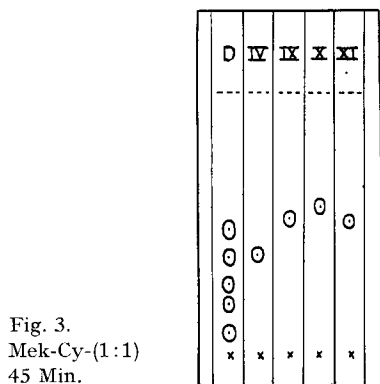
Fig. 1–4 sind Beispiele für Dünnschichtchromatogramme, schematisiert, aber massgetreu. Ausführung aufsteigend auf mit Kieselgel G «MERCK» beschichtetem Linienglas nach früheren Angaben [20]. Entwicklung mit p -Toluolsulfonsäure.
