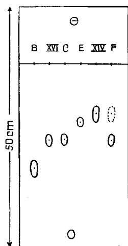
Fig. 1–4 sind Beispiele für Dünnschichtchromatogramme, schematisiert, aber massgetreu. Ausführung aufsteigend auf mit Kieselgel G «MERCK» beschichtetem Linienglas nach früheren Angaben [20]. Entwicklung mit p -Toluolsulfonsäure.
