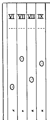
Fig. 1–4 sind Beispiele für Dünnschichtchromatogramme, schematisiert, aber massgetreu. Ausführung aufsteigend auf mit Kieselgel G «MERCK» beschichtetem Linienglas nach früheren Angaben [20]. Entwicklung mit p -Toluolsulfonsäure.
