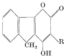
XIII: R = CH 2 C 6 H 5 XIV: R = H
