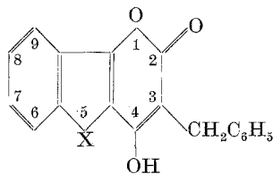
XI: X = O XII: X = S
