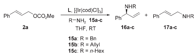
Scheme 17.
