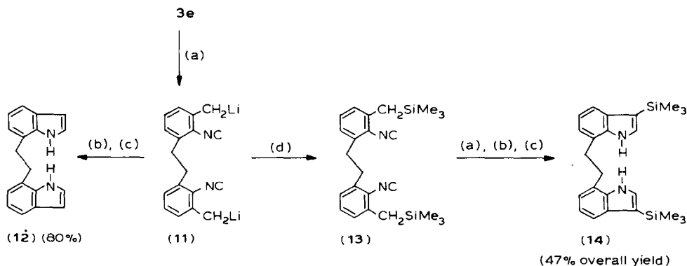
SCHEME 1. (a) 4LDA, -78^{\circ}\text{C} ; (b) -78^{\circ}\text{C} to r.t.; (c) \text{H}_2\text{O} ; (d) 4 \text{Me}_3\text{SiCl} .
