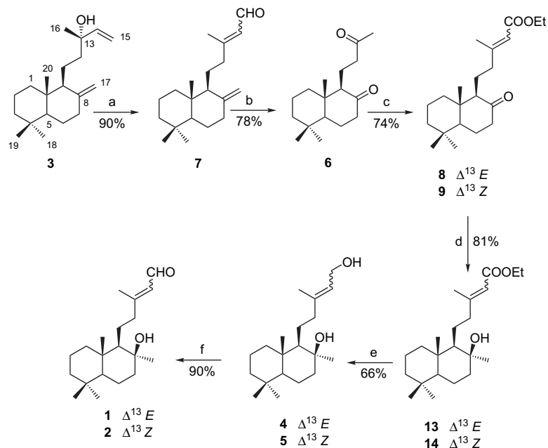
Scheme 1. (a) PCC, \text{CH}_2\text{Cl}_2 ; (b) (i) \text{O}_3 , \text{CH}_2\text{Cl}_2 , -78^\circ\text{C} ; (ii) \text{Ph}_3\text{P} , \text{CH}_2\text{Cl}_2 ; (c) triethylphosphonoacetate, NaH, THF, 0^\circ\text{C} ; (d) \text{MeMgCl} , \text{Et}_2\text{O} , -20^\circ\text{C} ; (e) LAH, THF, 0^\circ\text{C} ; (f) \text{MnO}_2 , \text{CH}_2\text{Cl}_2 .
