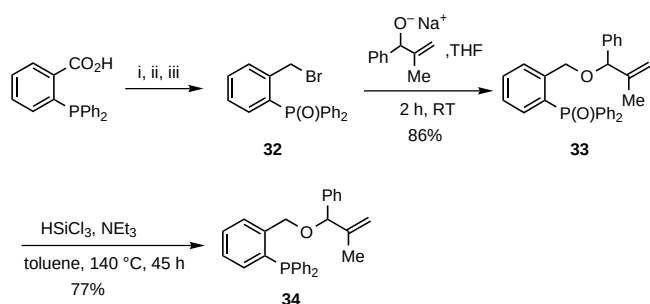
Scheme 7. Preparation of benzyl ether 34 : i) \text{LiAlH}_4 ; ii) \text{H}_2\text{O}_2 ; iii) \text{PBr}_3 .
