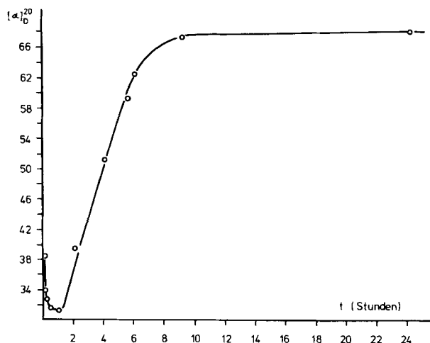
Fig. 2. Zeitliche Änderung des Drehwerts bei der Reaktion des Enolesters 5b ( \text{R}^6=\text{H} ) mit Leucin-methylester ( \text{CH}_2\text{Cl}_2 , 20^\circ , je 0,2M Lösungen): Bestimmung von t_2^8 )
