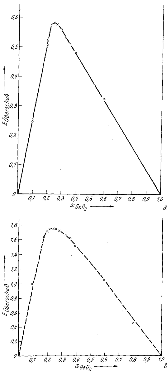
Abb. 5. Überschußextinktion in Abhängigkeit vom Molenbruch x_{\text{GeO}_2}
