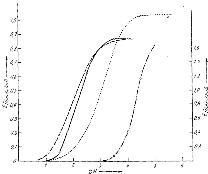
Abb. 4. Überschußextinktion in Abhängigkeit vom pH
