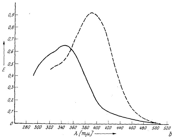
Abb. 3. a) Verschiebung des Absorptionsspektrums von 3-Nitrobenzocatechin in wäßriger Lösung durch Komplexbildung mit Germanium(IV) bei pH = 4,0
