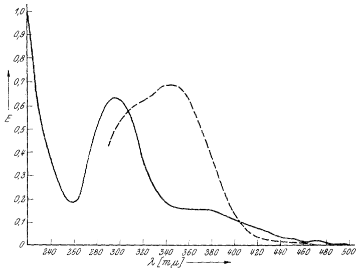
Abb. 2. Absorptionsspektren von 3-Nitrobrenzcatechin und 4-Nitrobrenzcatechin in wäßriger Lösung
