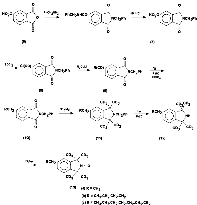
Scheme 2: Synthesis of 5-alkyl- ^{15}\text{N} -1,1,3,3-Tetrakis(trideuteriomethyl)isoindolin-2-ylxolyl
