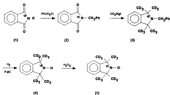
Scheme 1: Synthesis of ^{15}\text{N} -1,1,3,3-Tetrakis(trideuteriomethyl)isoindolin-2-ylxoyl
