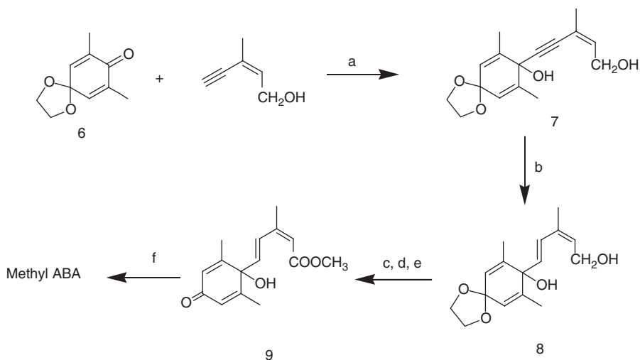
Scheme 2. Reagents (a) n -BuLi, THF; (b) Red-Al ® ; (c) MnO 2 , acetone; (d) MnO 2 , NaCN, AcOH, MeOH; (e) HCl, THF; (f) CH 3 MgBr
