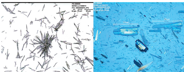
(b) IPA : H 2 O reslurry
