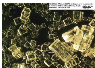
(a) EtOH: H 2 O 1: 1 recrystn.
