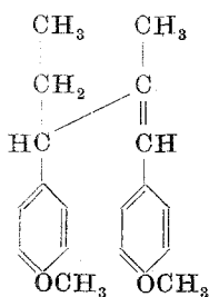
V Iso-anethol
