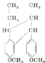
VI Meta-Anethol
