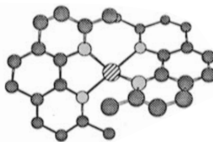
\text{Cu(dmp)}_2^{2+}
