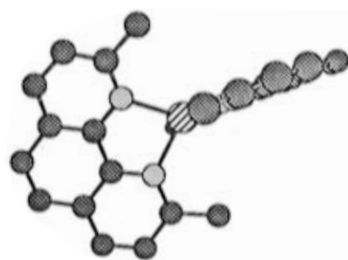
\text{Cu(dmp)}_2^+
