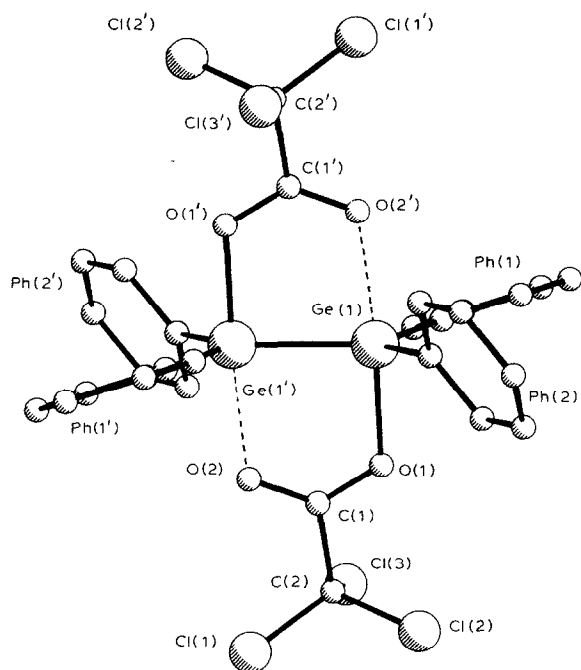
Fig. 1. Gefundenes 1,2-Bis(trichloroacetat)tetraphenyldigerman-Molekül (' zentrosymmetrisch ergänzte Atome, Ph(1) C(11) bis C(16), Ph(2) C(21) bis C(26)).
