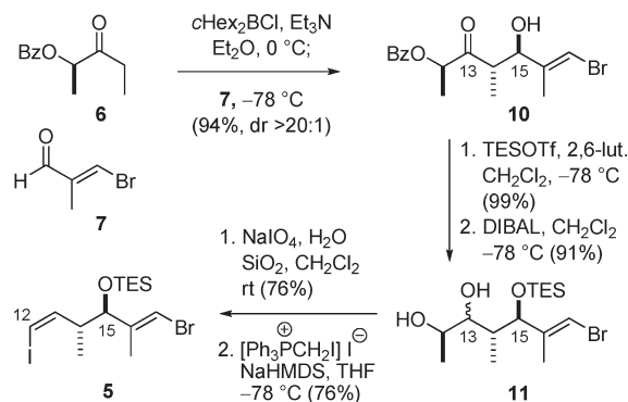
Scheme 2. Preparation of C12–C17 Bis -vinyl Halide 5
