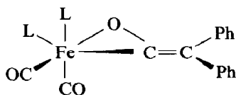
( 2d : L = P(OMe) 3 ; 2e : L = P(O- i -Pr) 3 )
