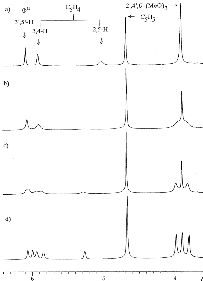
Fig. 1. ^1\text{H} -NMR spectra of 2a in \text{CDCl}_3 at (a) 25^\circ\text{C} , (b) -10^\circ\text{C} , (c) -20^\circ\text{C} , (d) -60^\circ\text{C} .
