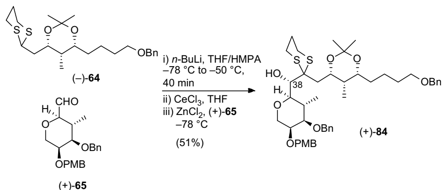
Scheme 30.
