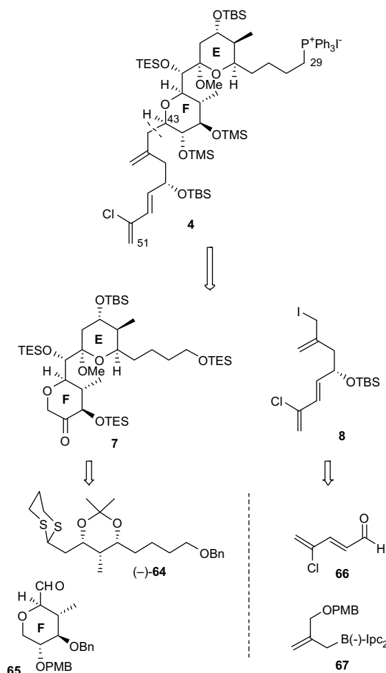
Scheme 24.
