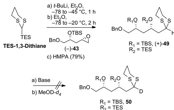
Scheme 16.
