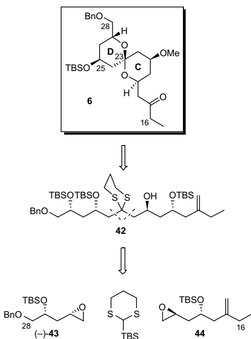
Scheme 14.
