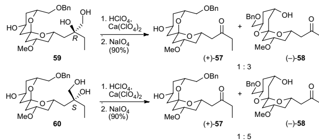
Scheme 21.
