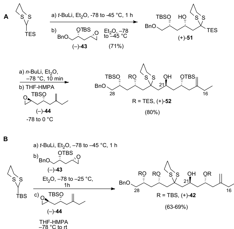
Scheme 17.
