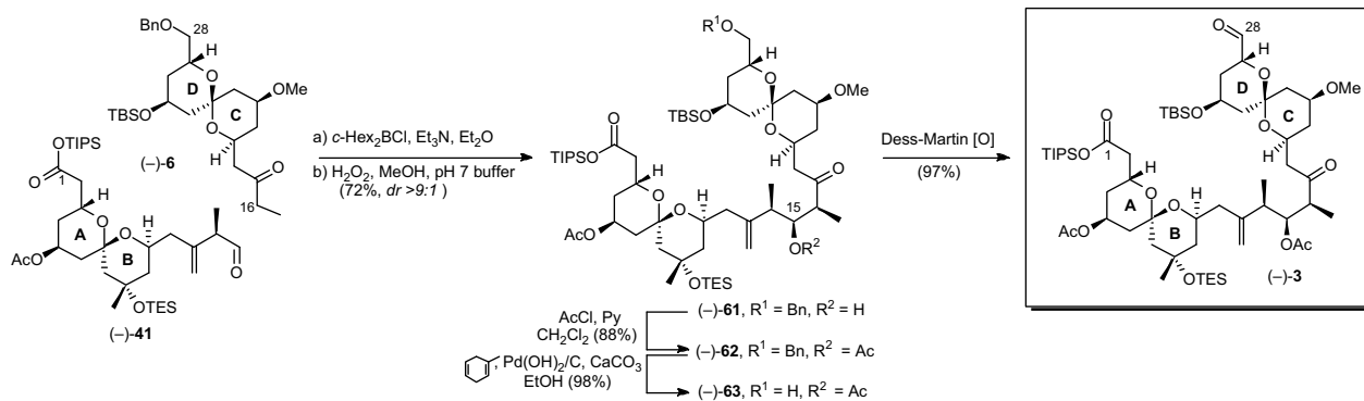
Scheme 23.
