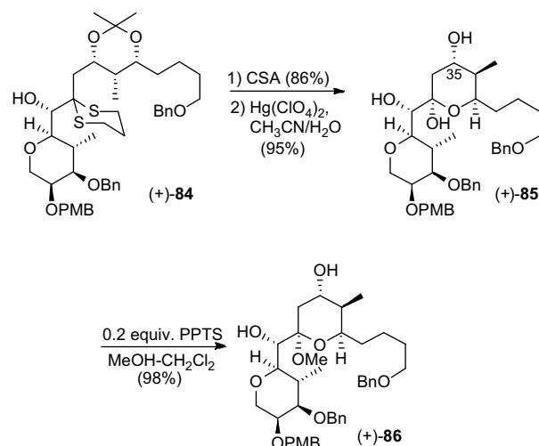
Scheme 31.
