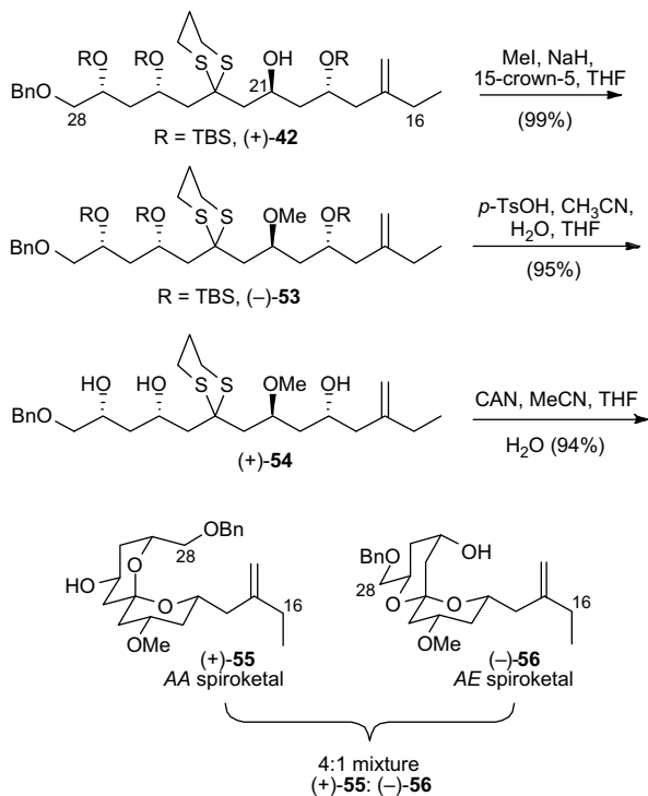
Scheme 18.
