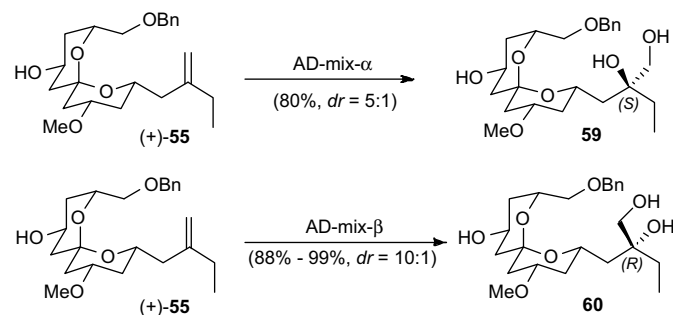
Scheme 20.
