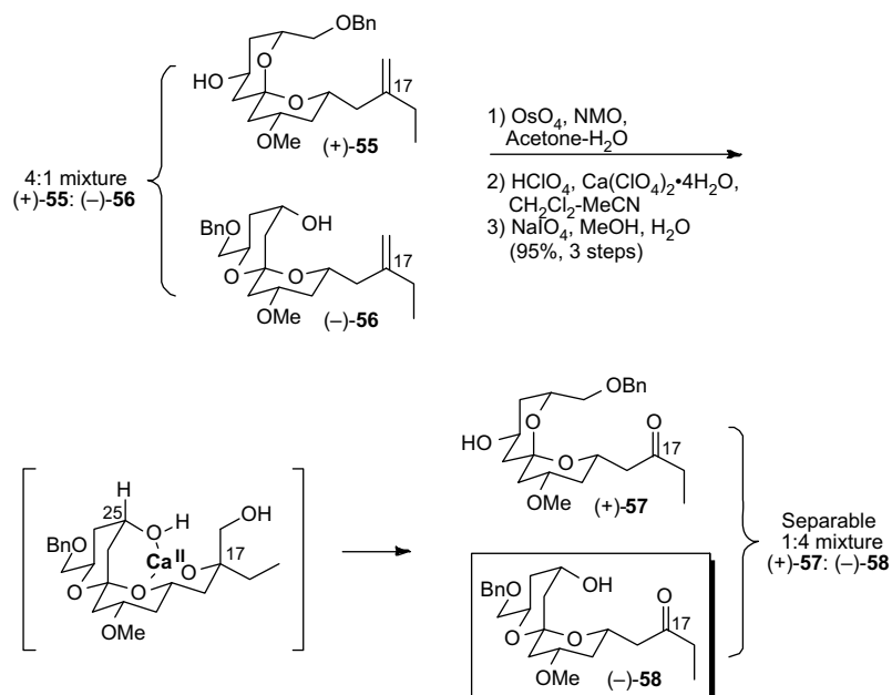
Scheme 19.
