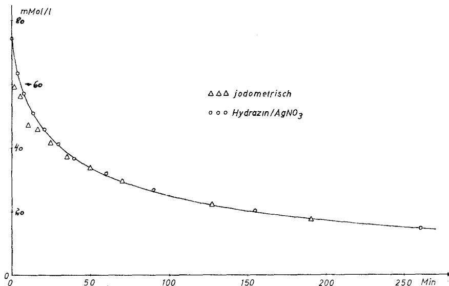
Abb. 5. Vergleich der jodometrischen Titrationsergebnisse mit den nach Abstopfung mit Eisessig—Hydrazin und potentiometrischer Bromtitration erhaltenen Werten
