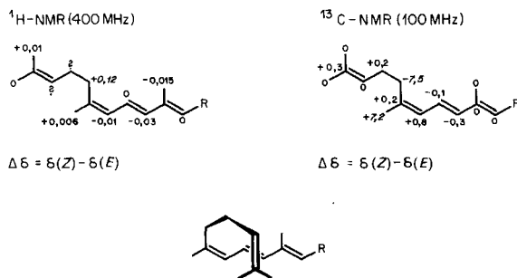
Fig. 2. Differenzen der chemischen Verschiebungen zwischen (5 E )- und (5 Z )- \psi -Endgruppe im ^1\text{H} - und ^{13}\text{C} -NMR-Spektrum; mögliche Konformation der (5 Z )- \psi -Endgruppe.
