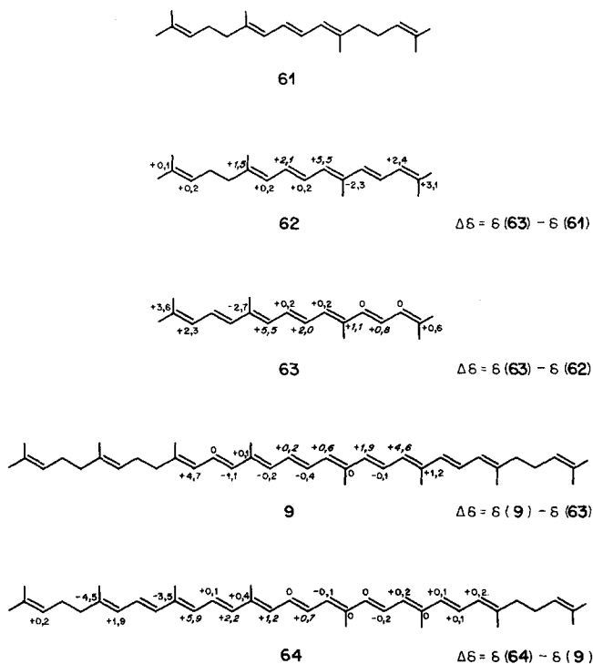
Fig. 1. Zur Zuordnung des ^{13}\text{C} -NMR-Spektrums von Neurosporin ( 9 )
