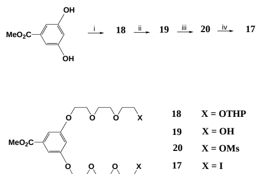
Scheme 6. Synthetic pathway to dielectrophile 17 : i) \text{Cl}(-\text{CH}_2-\text{CH}_2-\text{O})_3\text{-THP} , NaH, DMF; ii) pyridine \cdot HCl, EtOH; iii) MsCl, \text{Et}_3\text{N} , \text{CH}_2\text{Cl}_2 ; iv) NaI, acetone.
