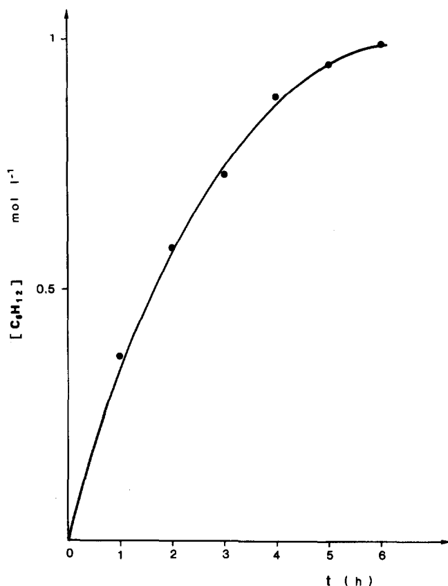
Fig. 1. Dimérisation du propylène catalysée par \text{HCo}(\text{COD})_2 ; P(\text{C}_3\text{H}_6) 5 bar; T 25°C; [\text{Co}]_0 0.1 mol l -1 .
