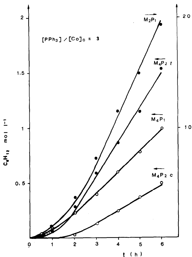
Fig. 4. Etude de la sélectivité. Concentration en dimères. [Co]_0 0.15\ mol\ l^{-1} ; T 25^\circ C ; P 3 bar; x = 3 .
