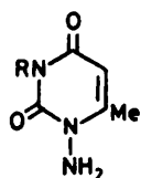
(5) R = H (6) R = Me
