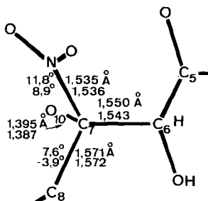
Fig. 4. Bindungslängen und Diederwinkel um C(7) von 17 (Der Wert für Molekel 17B steht jeweils unter dem für Molekel 17A)
