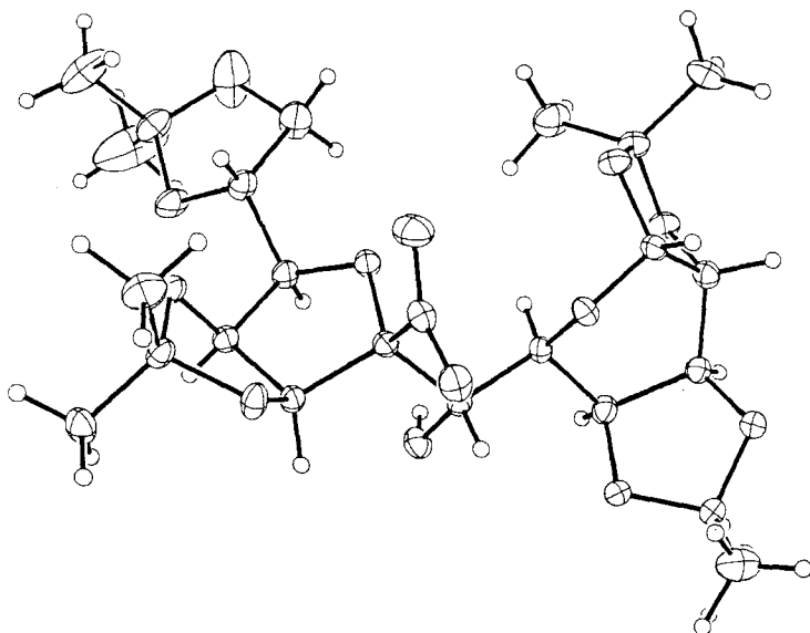
Fig. 2. Stereoprojektion einer der beiden symmetrieunabhängigen Molekeln 17A (Die H-Atome wurden mit willkürlichem Radius, die übrigen Atome mit thermischen Ellipsoiden für 50% Aufenthaltswahrscheinlichkeit dargestellt)
