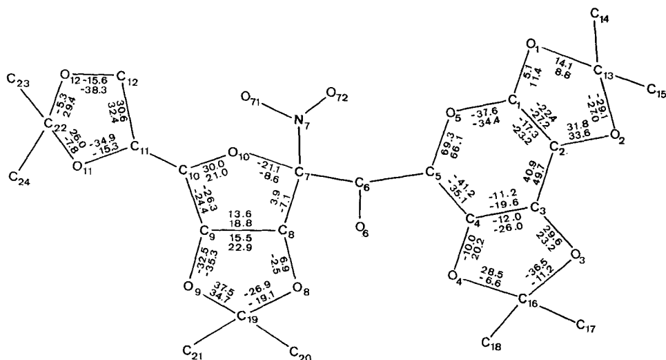
Fig. 1. Numerierung der Atome und intraannuläre Torsionswinkel (in Grad, Standardabweichungen 0,2–0,4°) von 17 (Der Wert für Molekel 17B steht jeweils unter dem für Molekel 17A )
