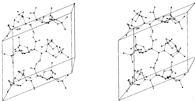
Fig. 3. Stereoskopisches Packungsdiagramm von 17 ohne die an C-Atome gebundenen H-Atome (Die H-Brücken sind gestrichelt wiedergegeben)
