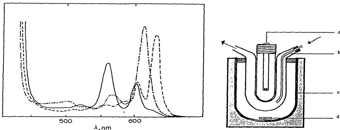
Fig. 1. Spectres visibles de la dihydroxystannyltétraphénylporphyrine et de ses formes réduites. — TPPSn(OH) 2 , \lambda_{\max} = 562 nm, \epsilon = 22000; ---- TPCSn(OH) 2 , \lambda_{\max} = 629 nm, \epsilon = 44300; - · - · - TPiBCSn(OH) 2 , \lambda_{\max} = 612 nm, \epsilon = 49900.
