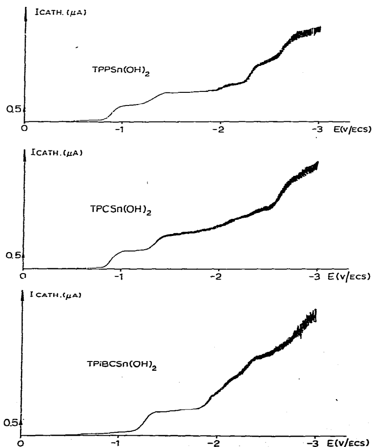
Fig. 3. Polarogrammes des réductions électrochimiques de TPPSn(OH) 2 ( 1.03 \times 10^{-3} M), TPCSn(OH) 2 ( 1.04 \times 10^{-3} M), TPiBCSn(OH) 2 ( 1.04 \times 10^{-3} M) dans THF 0.1 M en TBAP.
