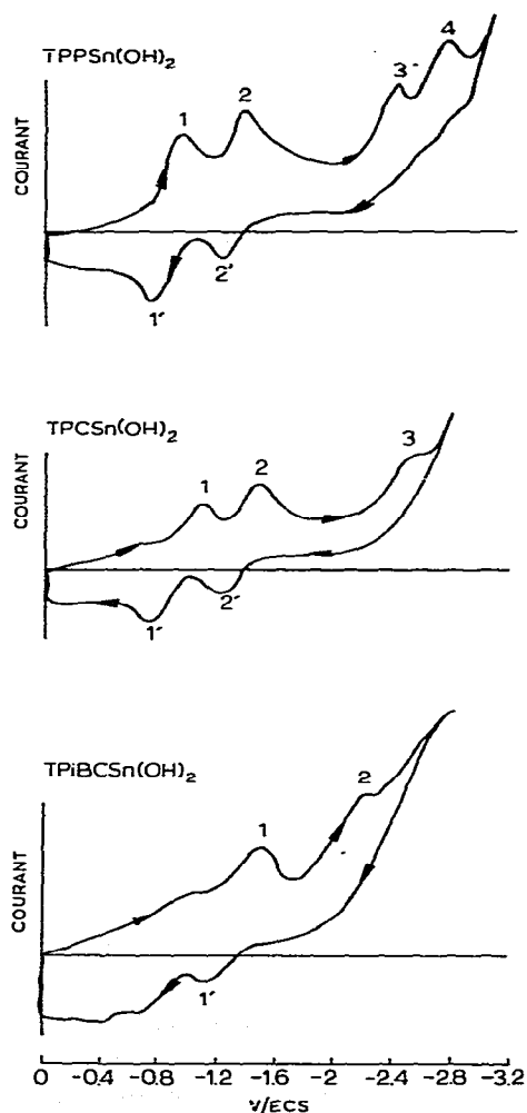
Fig. 4. Voltammétrie cyclique: réduction de \text{TPPSn(OH)}_2 ( 1.03 \times 10^{-3} M), \text{TPCSn(OH)}_2 ( 1.04 \times 10^{-3} M), \text{TPiBCSn(OH)}_2 ( 1.04 \times 10^{-3} M) dans THF + TBAP 0.1 M; 0 à -3.2 V/ECS; 160 \text{ mV s}^{-1} .
