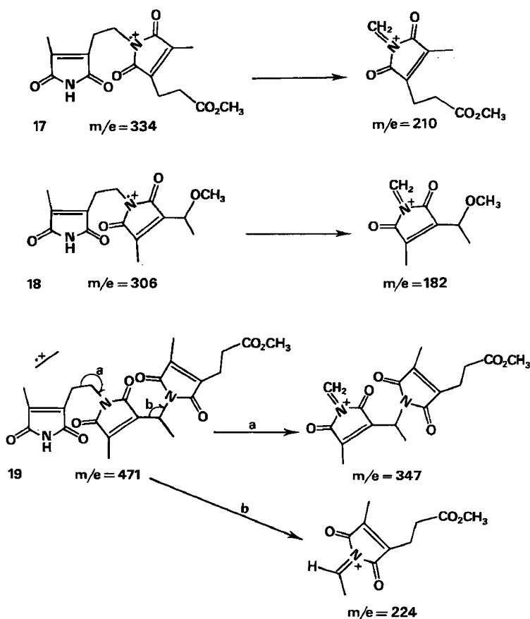
Schéma 3. Structures et fragmentations en spectrométrie de masse des produits d'oxydation particuliers aux esters de néobiliverdines: 17 produit d'oxydation de l'ester de néobiliverdine δ ( 16 ); 18 produit d'oxydation de l'ester de monométhoxydihydrophorcabiline ( 6 ); 19 produit d'oxydation de l'ester de l'isophorcabiline ( 7 )
