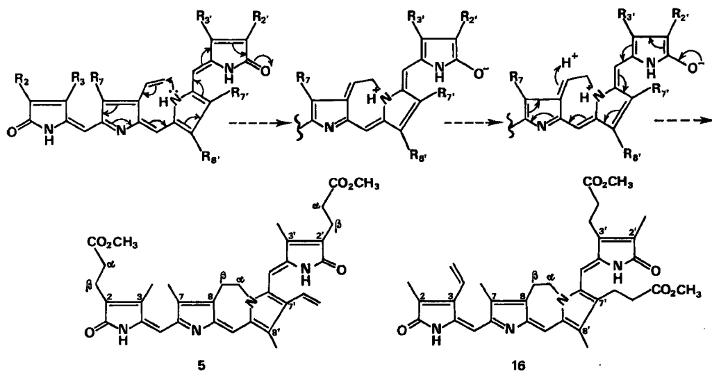
Schéma 4. Hypothèse de formation de la phorcabiline (5) à partir de ptérobiline ( R^3 = R^7 = R^{8'} = R^{3'} = \text{Me} ; R^{7'} = \text{V} ; R^2 = R^{2'} = \text{Pr} ), et de la néobiliverdine \delta (16) à partir de la biliverdine \delta ( R^2 = R^7 = R^{8'} = R^{3'} = \text{Me} ; R^3 = \text{V} ; R^{7'} = R^{3'} = \text{Pr} )
