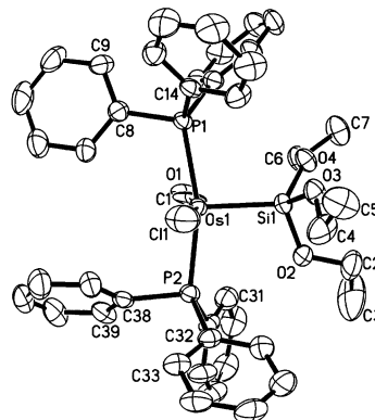
Fig. 1. Molecular geometry of Os[Si(OEt) 3 ]Cl(CO)(PPh 3 ) 2 ( 1 ).
