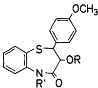
(+) - and (-) - 6 R R' (+) - and (-) - 7 H H (-) - 1 - [2 R ,3 R ] CH 3 CO CH 2 CH 2 N(CH 3 ) 2 CH 2 CH 2 N(CH 3 ) 2 · HCl
