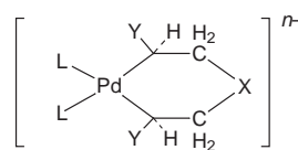
10a X = OC(=O)O 10b X = O
