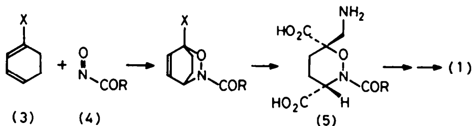
Scheme 1. E.g. R = OCH 2 Ph ; X = CO 2 Et
