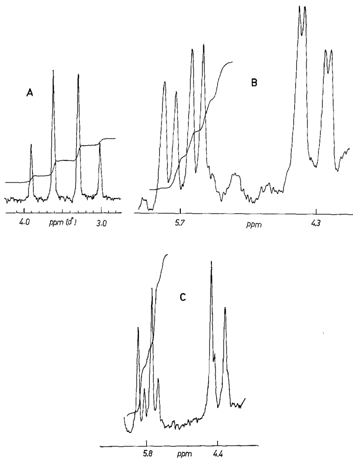
Abb. 4. NMR-Spektren von 2 im Gebiet der Benzyl-protonen. A: racem. 2 ; B und C: racem. 2 und (—)- 2 ( -107^\circ ) mit Zusatz von etwa 3–4fach molarem Überschuß von chiralem -Reagens, „shift“ (CAT-Spektren)
