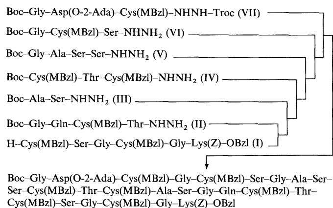
Fig. 2. Synthetic Scheme for A. bisporus Metallothionein
