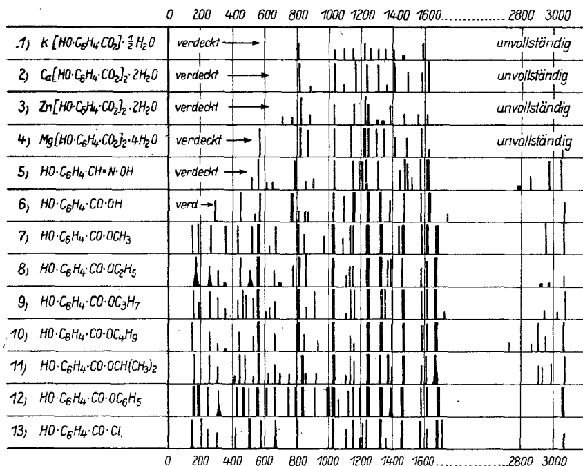
Fig. 1. Nr. 1—4 salicylsäure Salze, Nr. 5 Salicylaldoxim, Nr. 6 Salicylsäure. Nr. 1—6 Kristallpulveraufnahmen, Nr. 7—11 Alkylester. Nr. 12 Phenylester (Salol), Nr. 13 Salicoylchlorid. Nr. 7—13 Flüssigkeitsaufnahmen.
