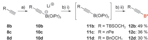
Scheme 3. a) i) n BuLi, Et 2 O, –78°C; ii) B(O i Pr) 3 ; b) i) 1.33 equiv BF 3 ·Et 2 O, THF, –78°C; ii) diol 1 , THF, –78°C → RT.
