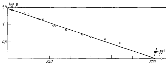
Fig. 1. Dampfdruck des o-Nitrobenzaldehyd.
