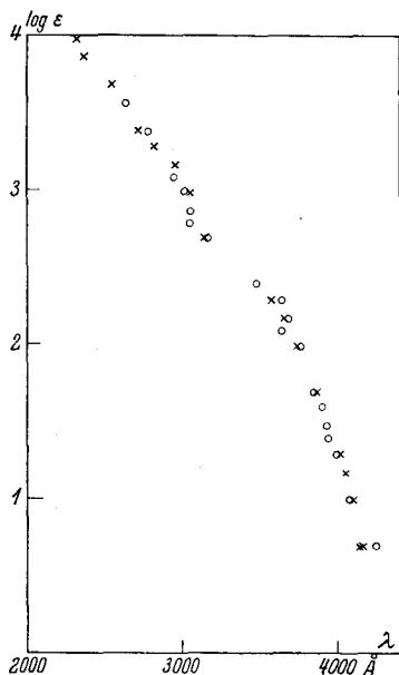
Fig. 2. Extinktion des o-Nitrobenzaldehyds in Alkohol (o) und in Hexan (x).
