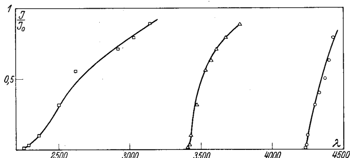
Fig. 4. Durchlässigkeit bei 1\text{ cm} Schichtdicke.
